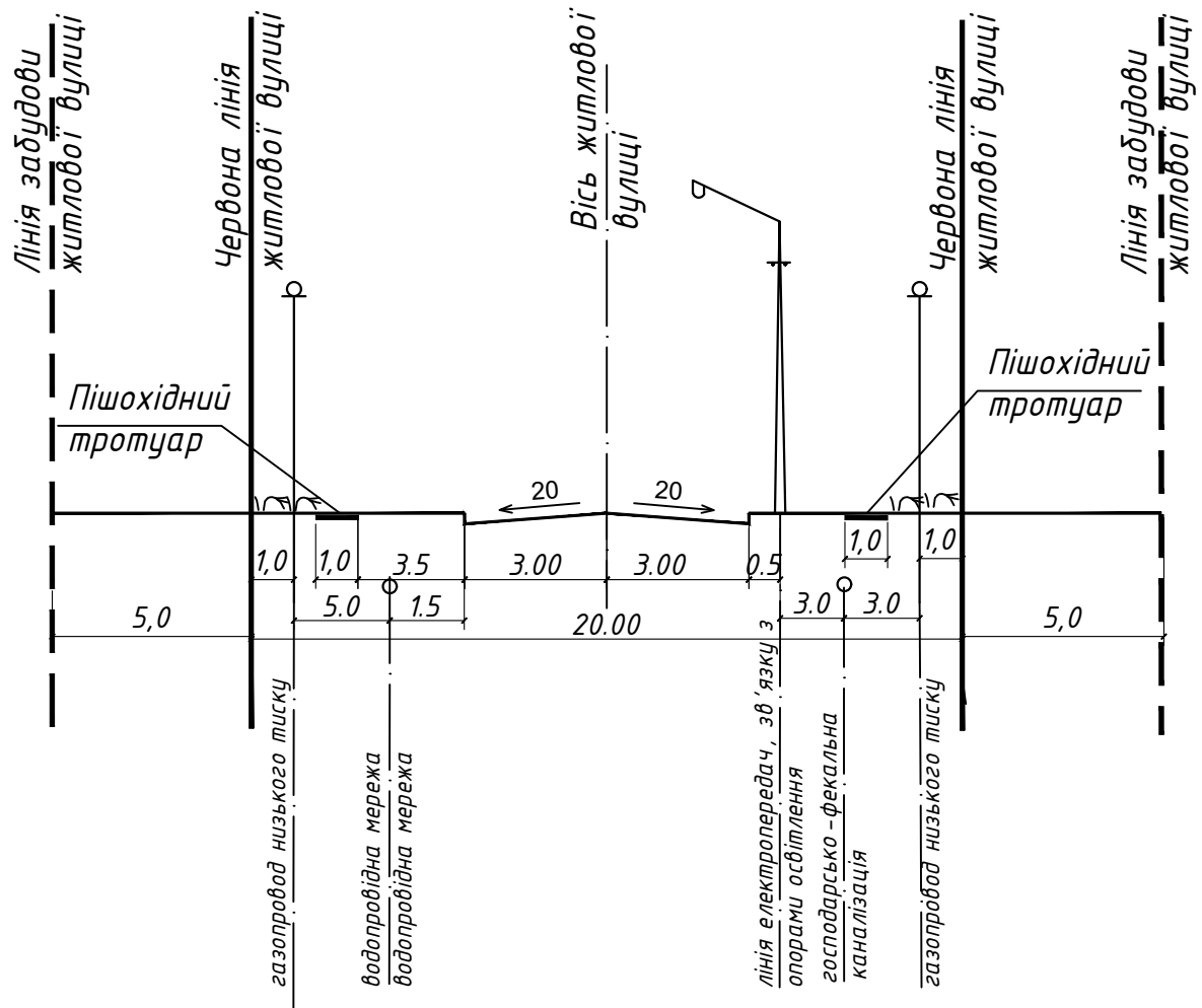
Розрахунок параметри житлової вулиці
